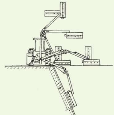
Schlegelmulcher
