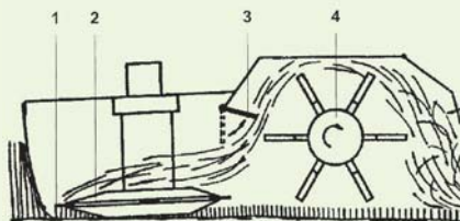
Trommelmäher (mit Aufbereiter)
